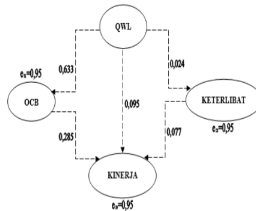
Gambar 1. Diagram Analisis Jalur
