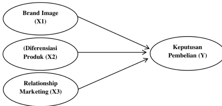
Gambar 1. Kerangka Pemikiran
